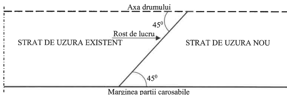
Fig. 1 Racordarea in plan a stratului nou cu stratul existent
