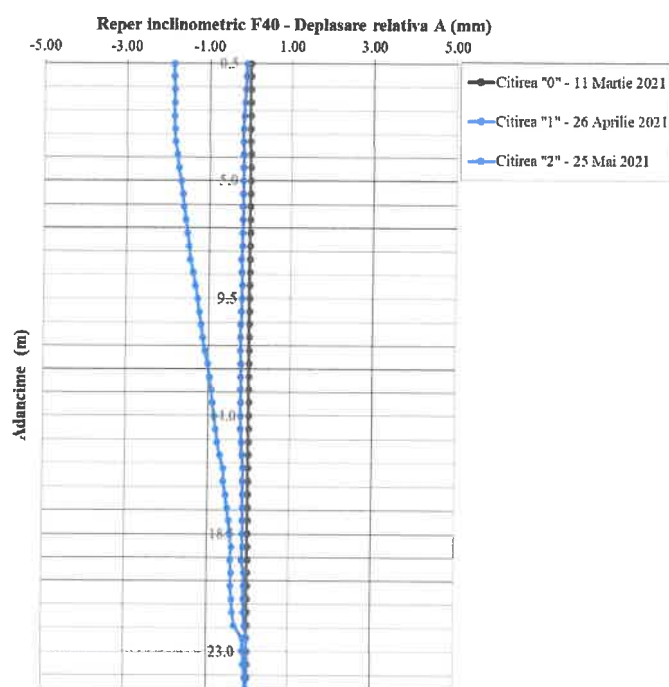
Fig. 3.45: Reper inclinometric F40 – Direcția A0-A180
