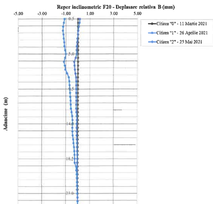
Fig. 3.22: Reper inclinometric F20 – Direcția B0-B180
