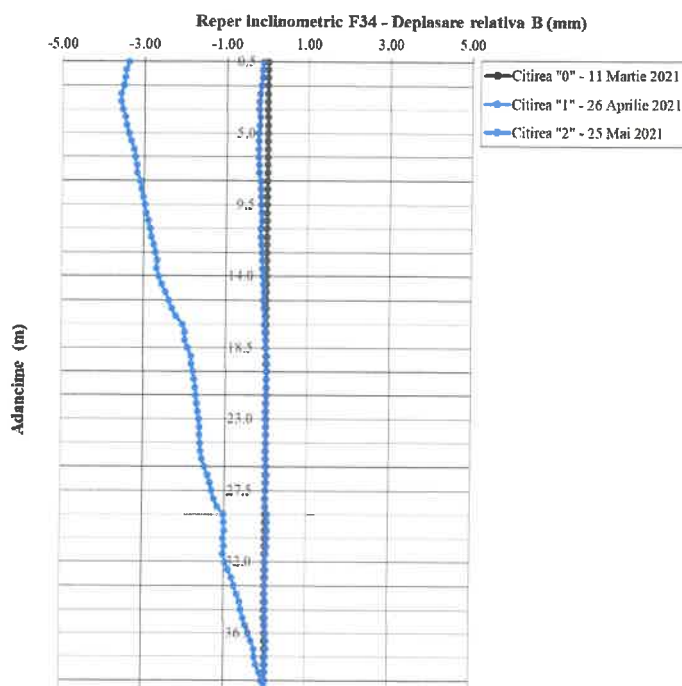
Fig. 3.28: Reper inclinometric F34 – Direcția B0-B180
