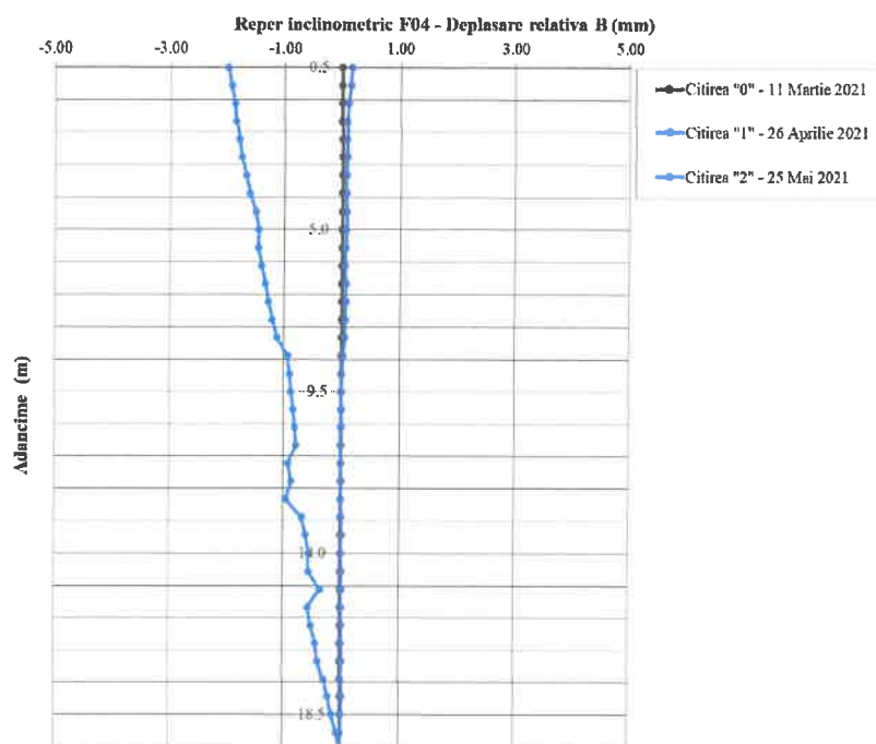
Fig. 3.4: Reper inclinometric F04 – Direcția B0-B180
