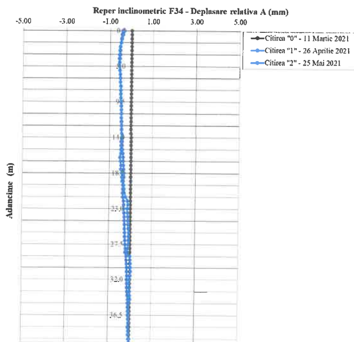
Fig. 3.27: Reper inclinometric F34 – Direcția A0-A180
