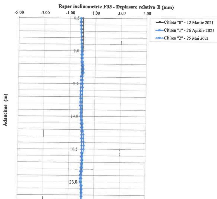
Fig. 3.25: Reper inclinometric F33 – Direcția B0-B180
