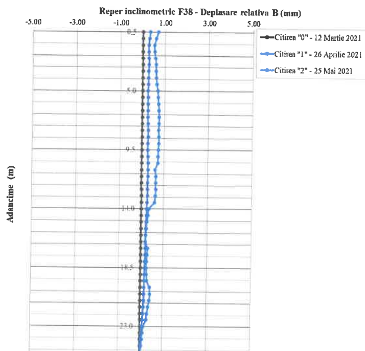
Fig. 3.40: Reper inclinometric F38 – Direcția B0-B180
