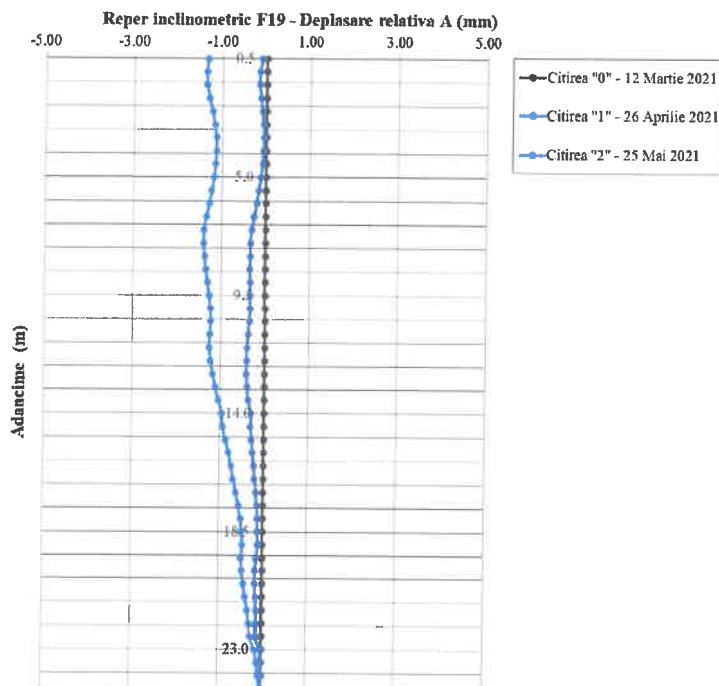
Fig. 3.18: Reper inclinometric F19 – Direcția A0-A180
