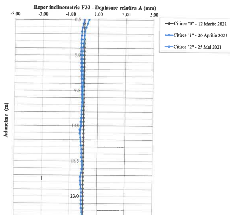
Fig. 3.24: Reper inclinometric F33 – Direcția A0-A180
