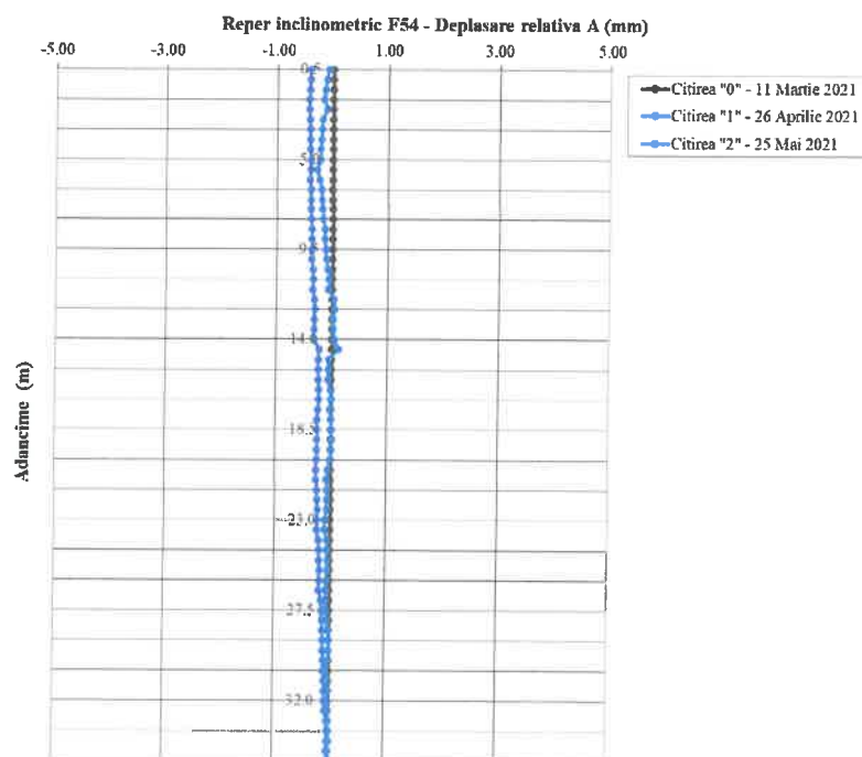
Fig. 3.51: Reper inclinometric F54 – Direcția A0-A180
