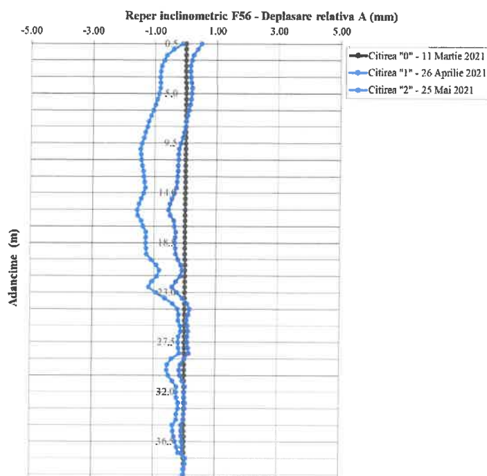
Fig. 3.54: Reper inclinometric F56 – Direcția A0-A180
