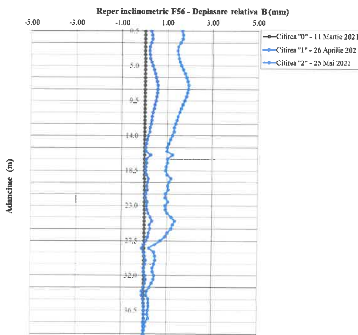
Fig. 3.55: Reper inclinometric F56 – Direcția B0-B180
