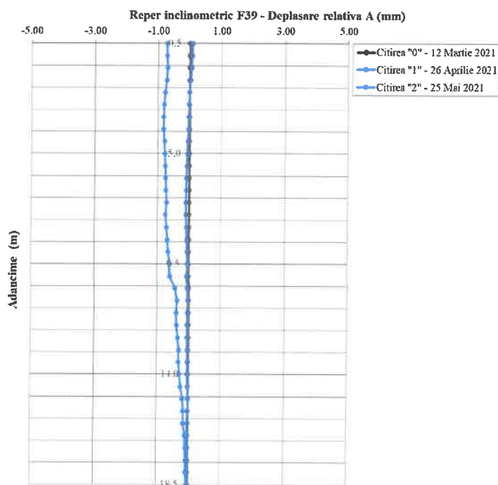
Fig. 3.42: Reper inclinometric F39 – Direcția A0-A180
