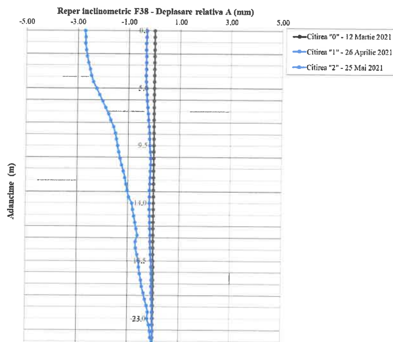
Fig. 3.39: Reper inclinometric F38 – Direcția A0-A180
