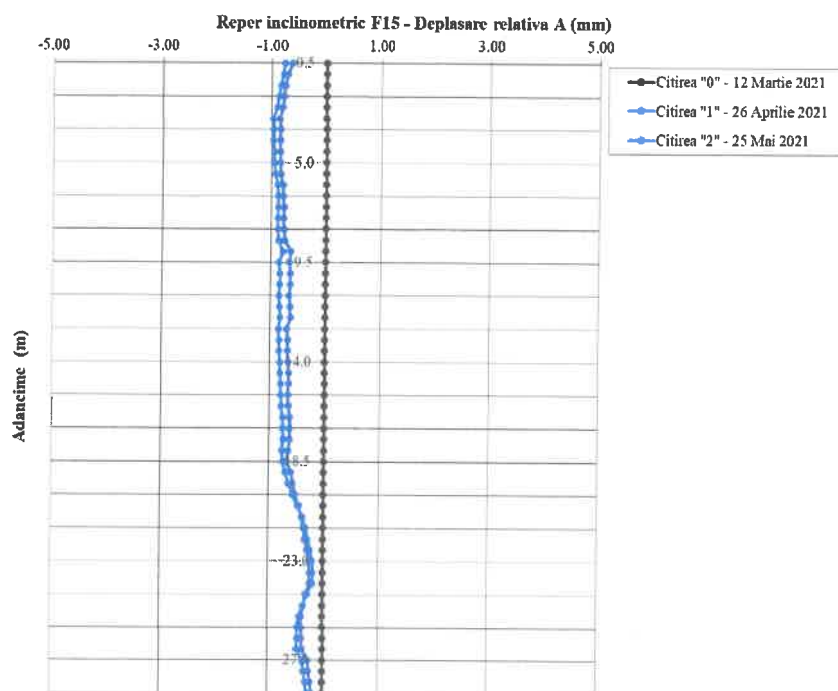
Fig. 3.12: Reper inclinometric F15 – Direcția A0-A180
