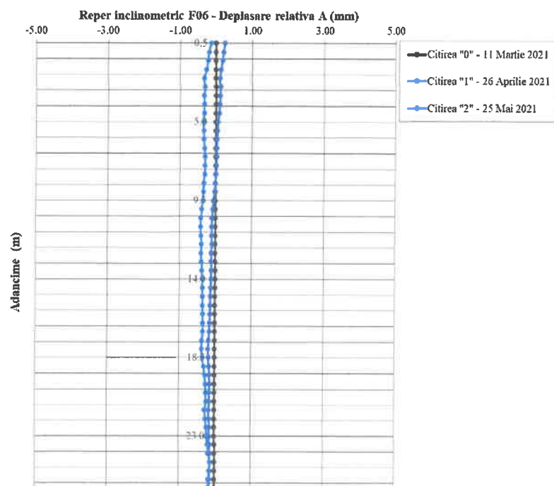
Fig. 3.6: Reper inclinometric F06 – Direcția A0-A180
