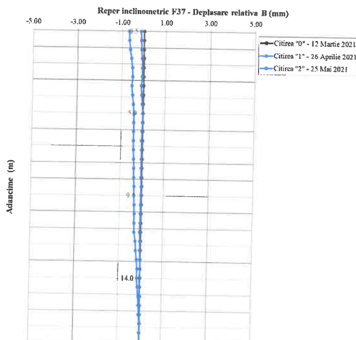
Fig. 3.37: Reper inclinometric F37 – Direcția B0-B180
