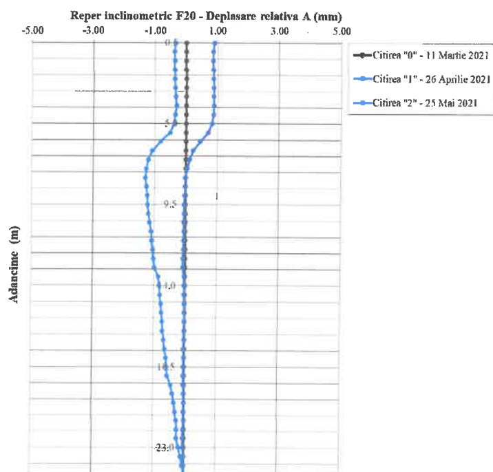
Fig. 3.21: Reper inclinometric F20 – Direcția A0-A180
