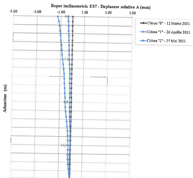
Fig. 3.36: Reper inclinometric F37 – Direcția A0-A180
