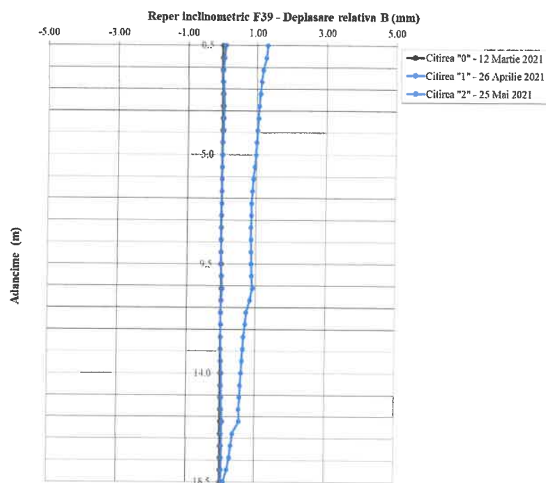
Fig. 3.43: Reper inclinometric F39 – Direcția B0-B180
