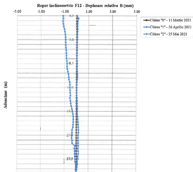
Fig. 3.10: Reper inclinometric F12 – Direcția B0-B180
