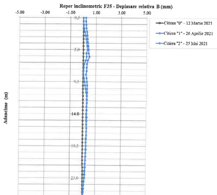
Fig. 3.31: Reper inclinometric F35 – Direcția B0-B180
