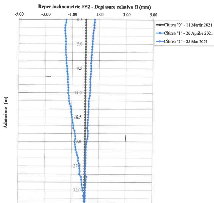
Fig. 3.49: Reper inclinometric F52 – Direcția B0-B180
