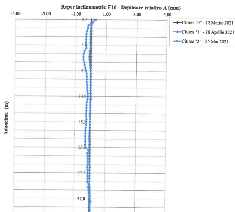
Fig. 3.15: Reper inclinometric F16 – Direcția A0-A180
