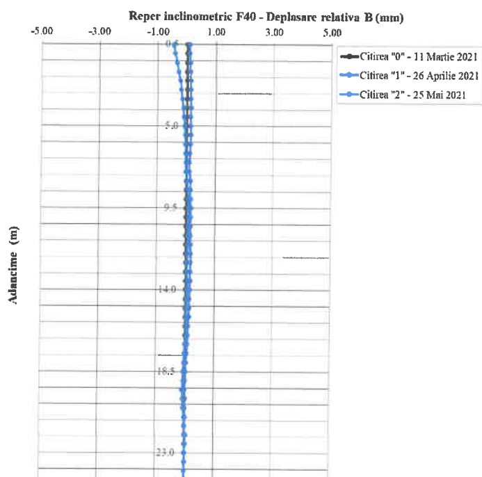
Fig. 3.46: Reper inclinometric F40 – Direcția B0-B180
