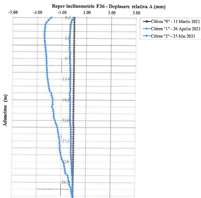
Fig. 3.33: Reper inclinometric F36 – Direcția A0-A180
