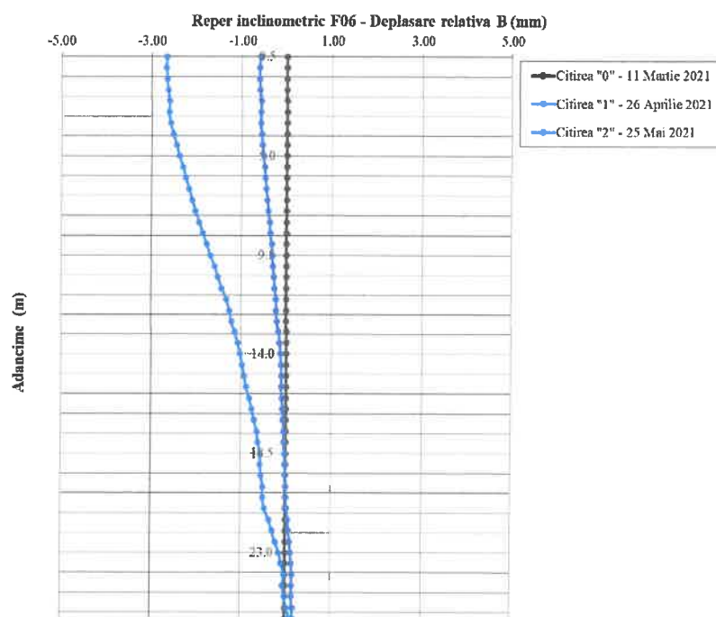
Fig. 3.7: Reper inclinometric F06 – Direcția B0-B180
