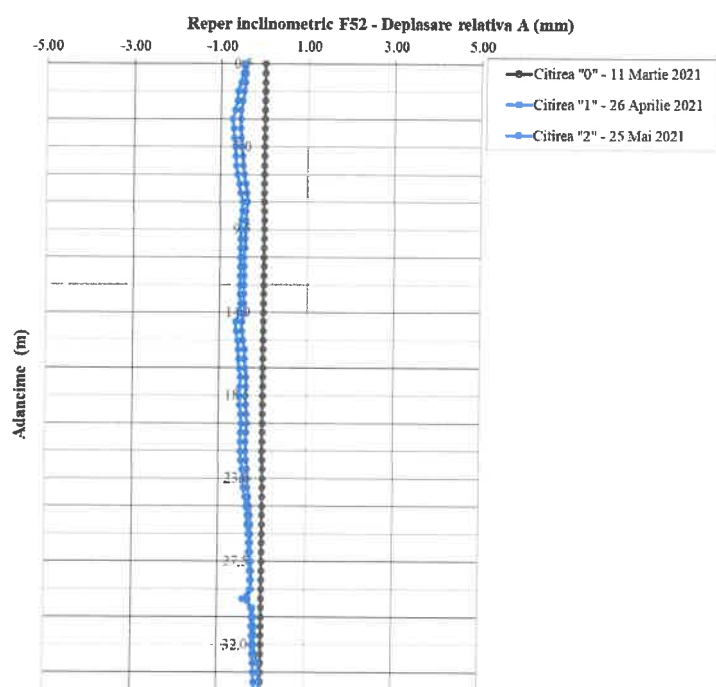
Fig. 3.48: Reper inclinometric F52 – Direcția A0-A180
