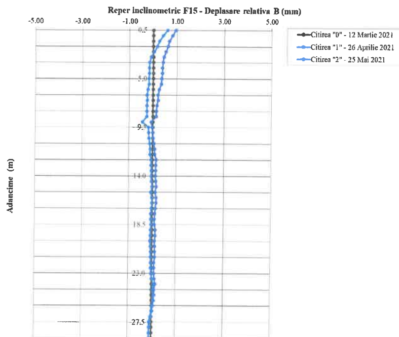
Fig. 3.13: Reper inclinometric F15 – Direcția B0-B180
