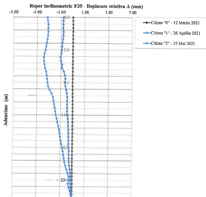
Fig. 3.30: Reper inclinometric F35 – Direcția A0-A180
