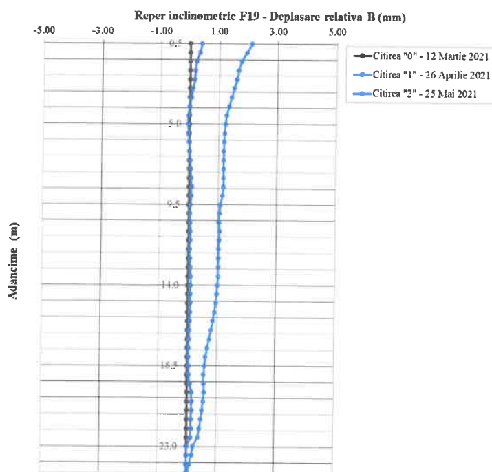
Fig. 3.19: Reper inclinometric F19 – Direcția B0-B180
