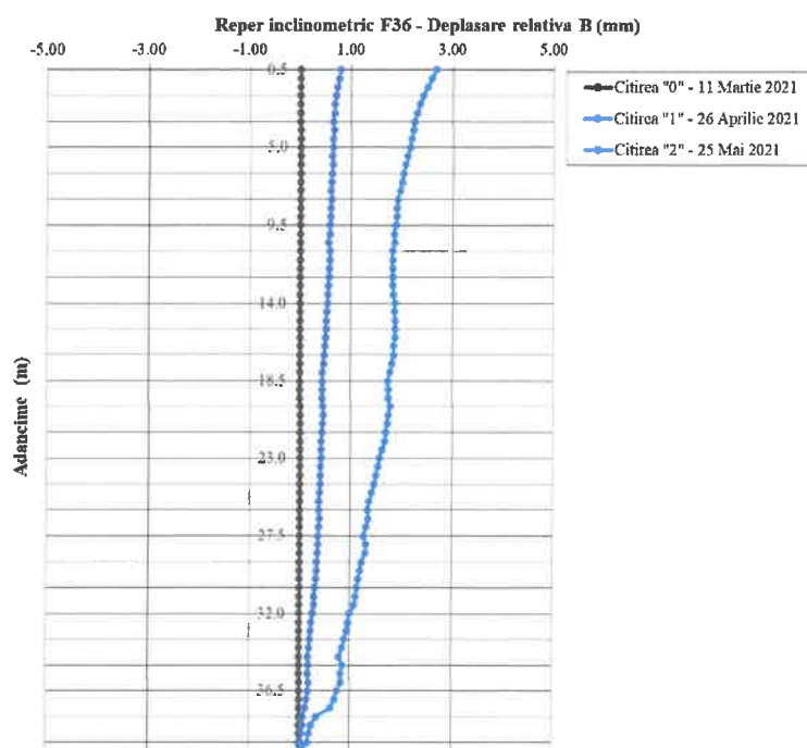
Fig. 3.34: Reper inclinometric F36 – Direcția B0-B180
