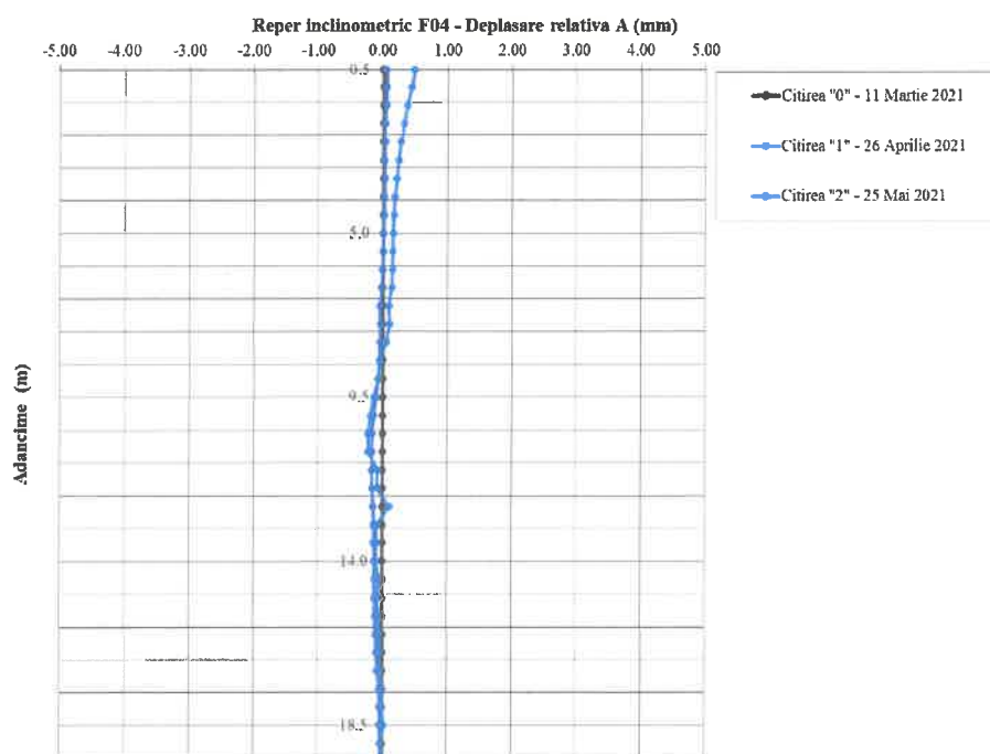
Fig. 3.3: Reper inclinometric F04 – Direcția A0-A180
