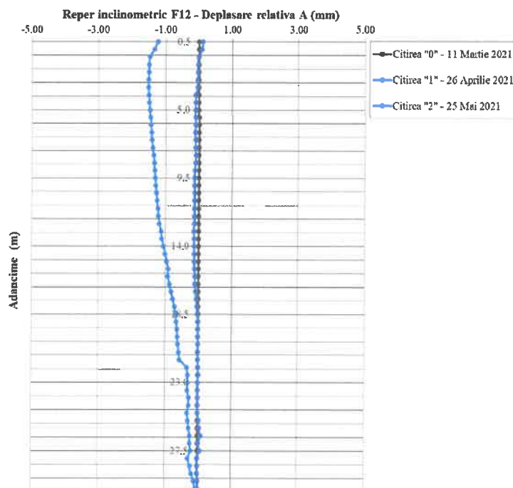
Fig. 3.9: Reper inclinometric F12 – Direcția A0-A180
