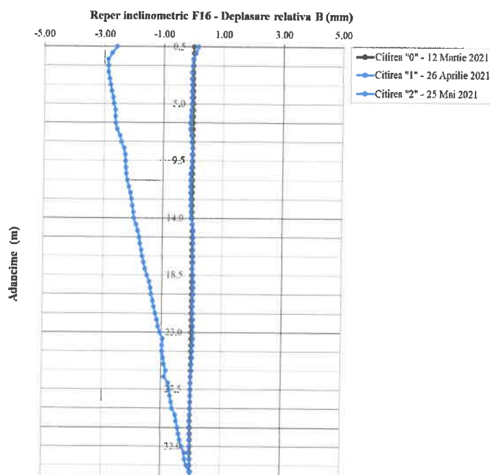
Fig. 3.16: Reper inclinometric F16 – Direcția B0-B180
