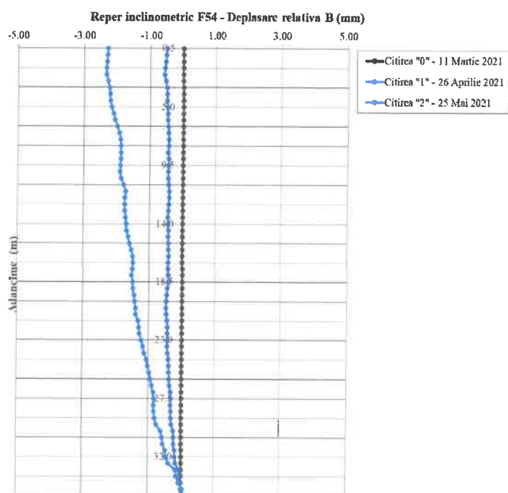
Fig. 3.52: Reper inclinometric F54 – Direcția B0-B180
