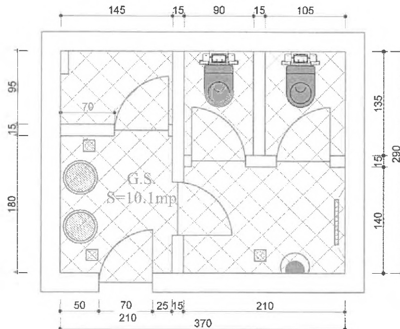
G.S. Etaj 2 - Drumuri B propus (12)
