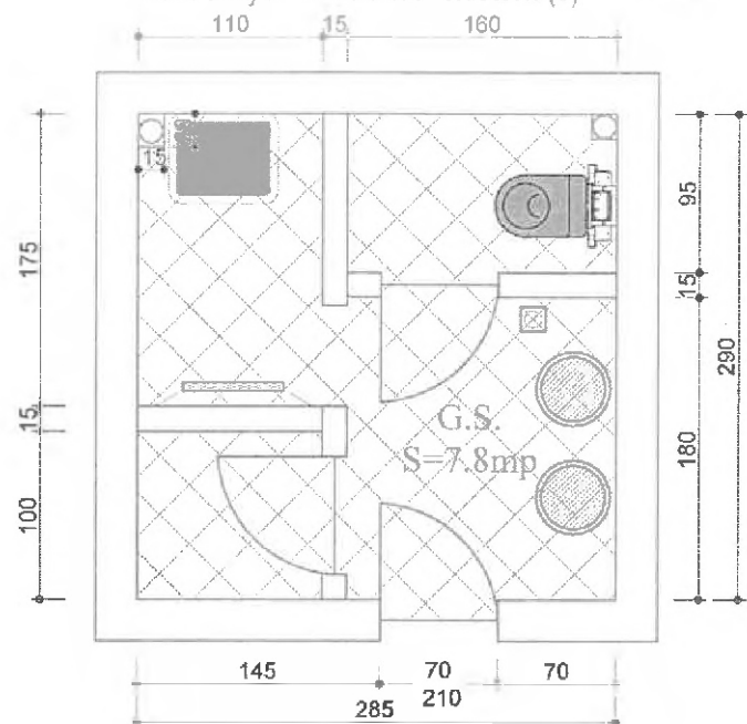
G.S. Etaj 2 - Drumuri F existent (8)
