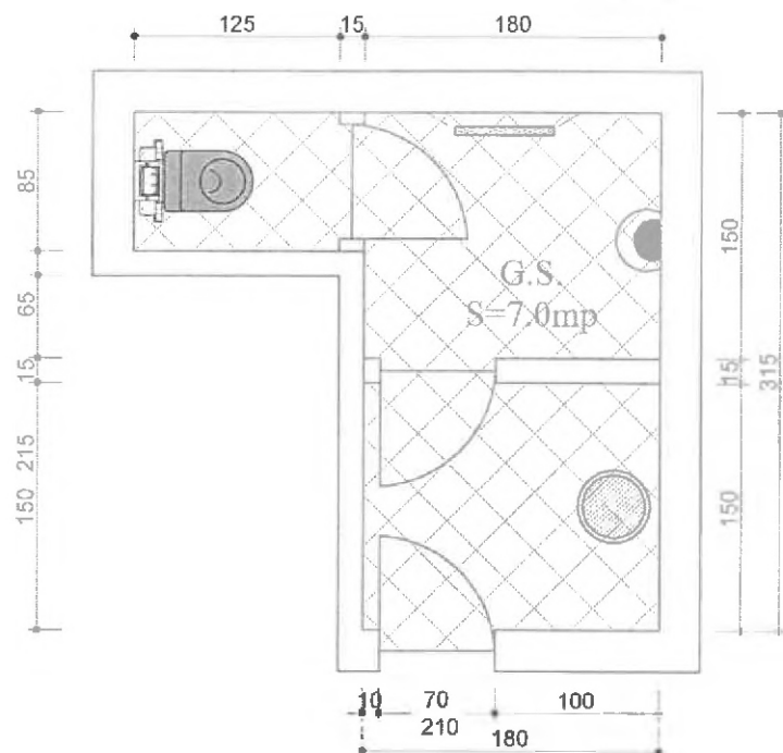
G.S. Etaj 1 - IT B (6)
