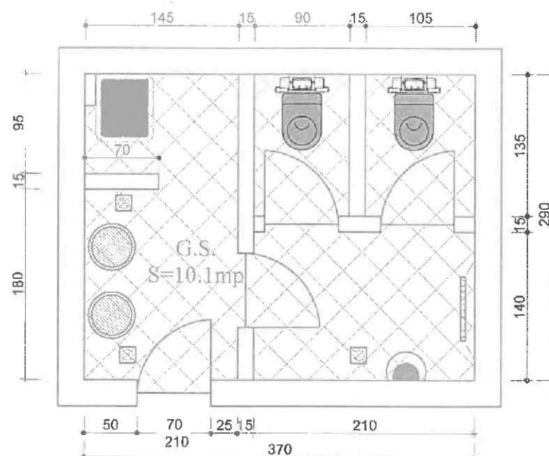
G.S. Etaj 2 - Drumuri B existent (12)
