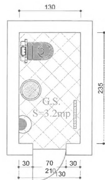
G.S. Mansarda - SCIM B (11)
