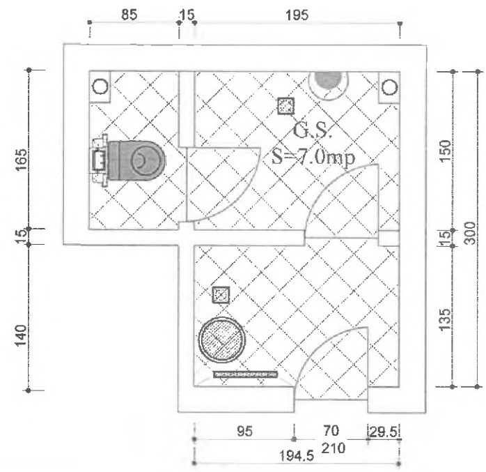
G.S. Etaj 1 - Juridic B (13)
