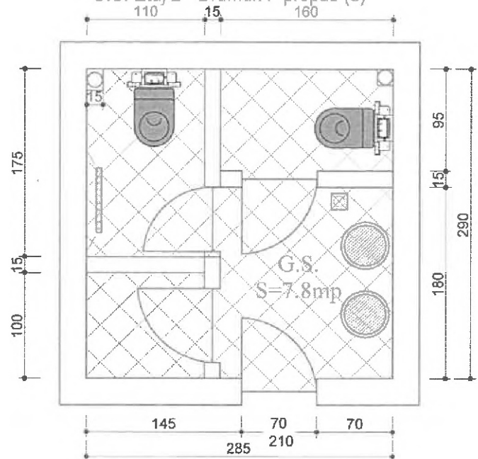
G.S. Etaj 2 - Drumuri F propus (8)
